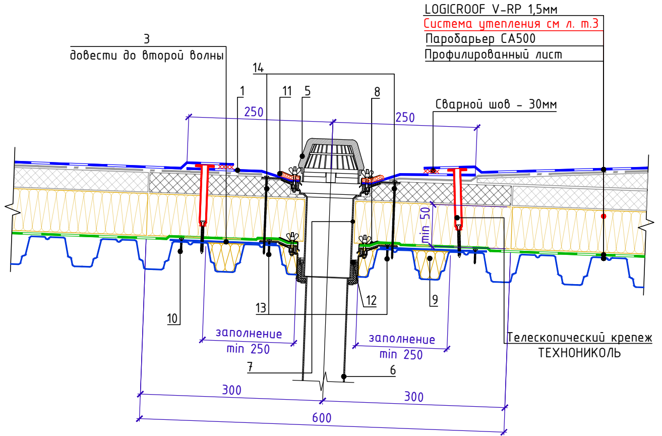
Спецификация на узел У.2.3-2020.07
