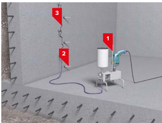
1. Электрический поршневой насос; 2. Инъекционные пакеры; 3. Трещина или технологический шов бетонирования.
