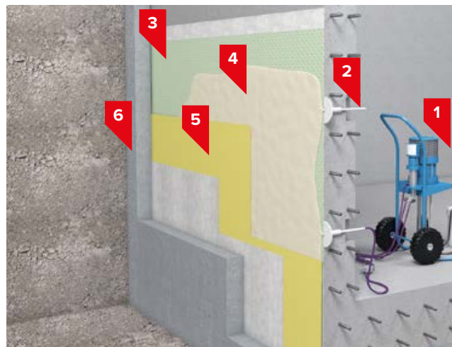
Б.) Инъектирование двухслойной системы гидроизоляции
