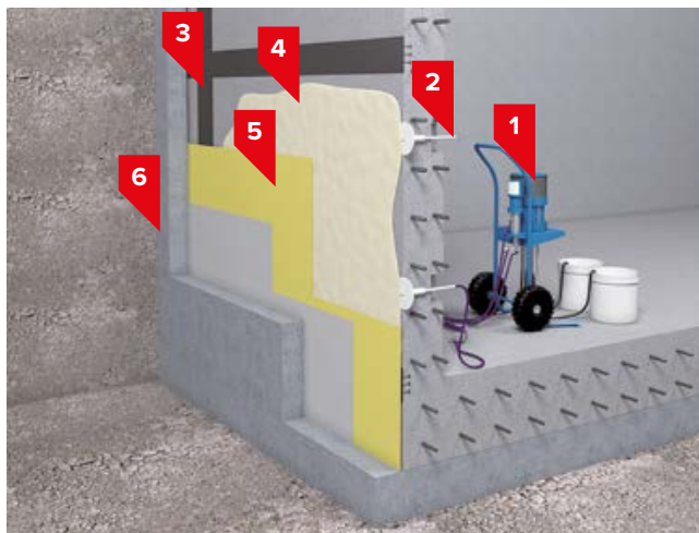
А.) Инъектирование однослойной системы гидроизоляции
