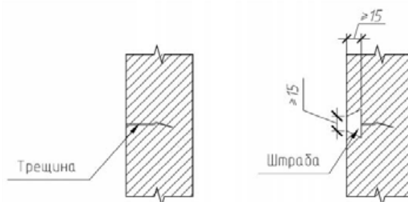
Рисунок 8.1 – Схема выполнения штрабы
