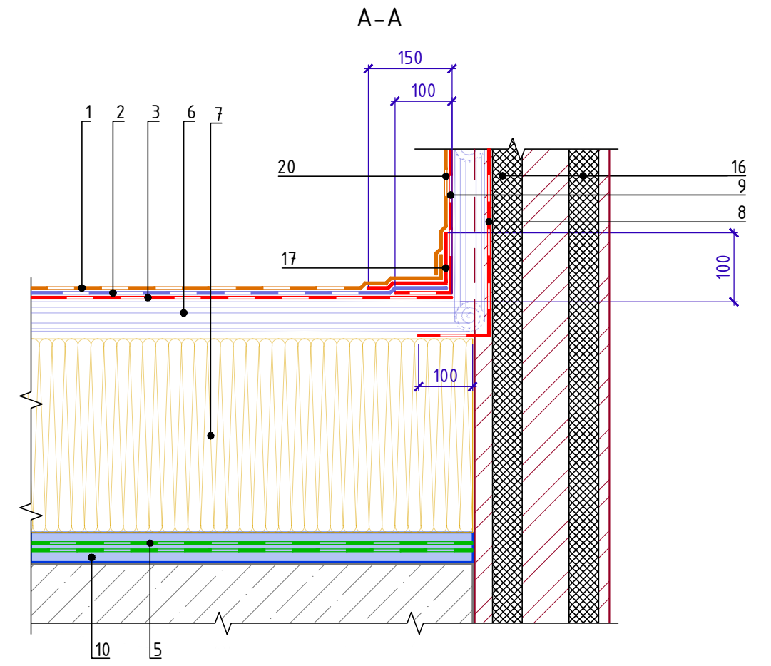
Спецификация на узел У.6.1-2021.12
