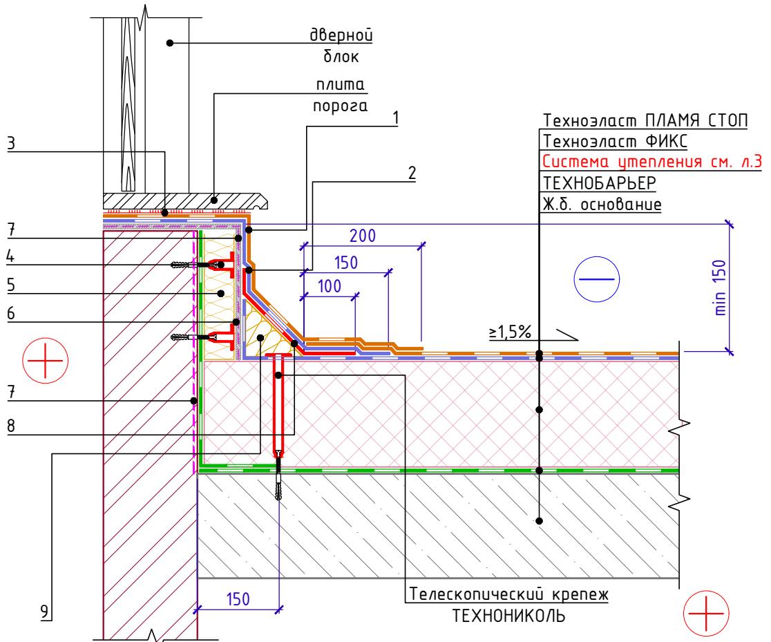
Спецификация на узел Ч.9.1-2020.09
