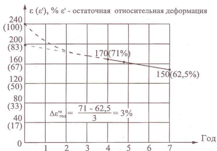
Рис.3. Изменение относительной (остаточной относительной) деформации материала “Loqicroof V-RP 1.2” при старении в кровельном ковре в натуральных условиях
