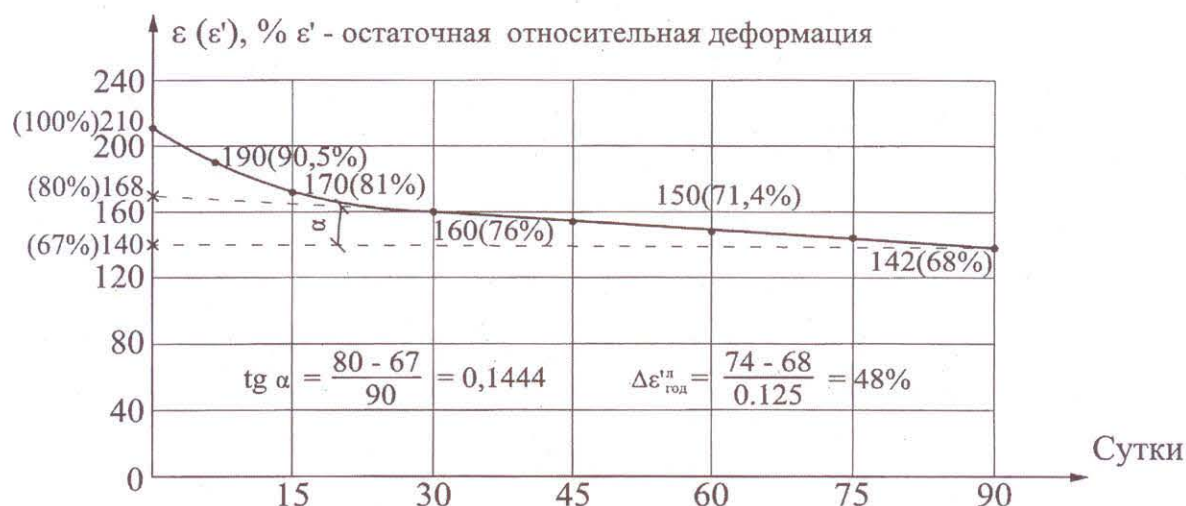
Рис. 1. Изменение относительной (остаточной относительной) деформации материала “Loqicroof V-RP 1.2” при термостарении в лабораторных условиях.
