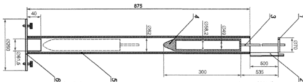
1 - упор; 2 - съемный упор; 3 - штанга; 4 - груз; 5 - труба; 6 - опорная площадка
