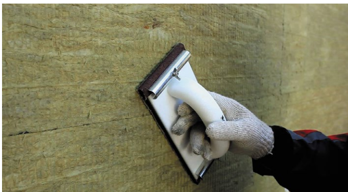
Рис. 12. Шлифовка стыков плит теплоизоляции наждачной бумагой
