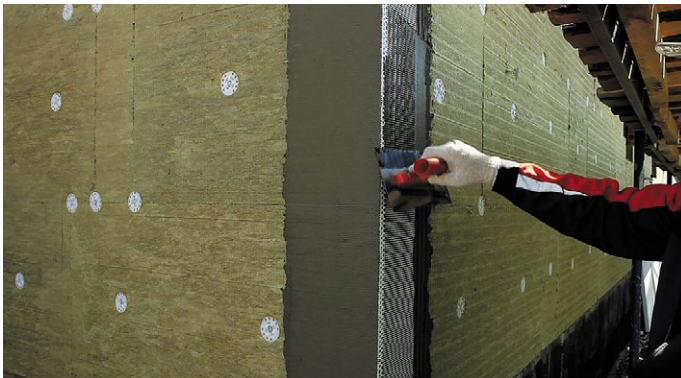
Рис. 15. Установка усиливающих профилей на углах здания
