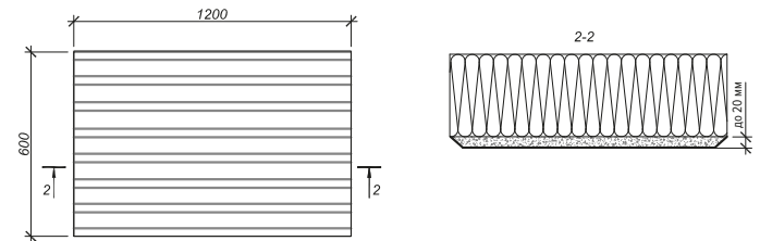
Рис. 5. Схема сплошного нанесения клея на плиту
