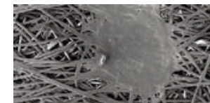
Структура иглопробивного геотекстиля типа спанбонд
