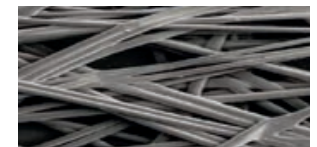
Структура геотекстиля «Тураг». Однородность структуры по всему полотну определяет отсутствие мест с высокой плотностью, хуже пропускающих воду
