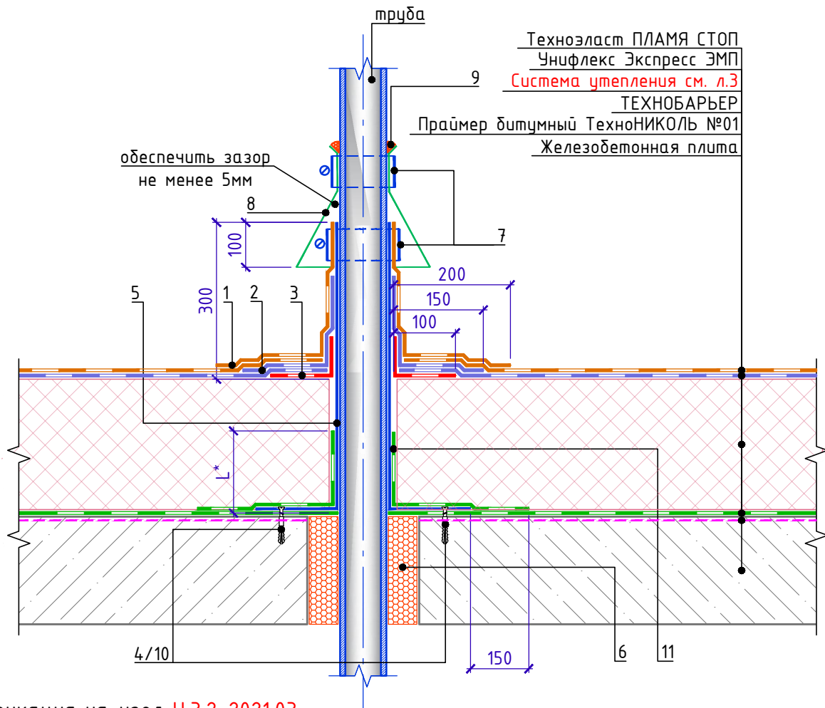
Спецификация на узел У.3.2-2021.03
