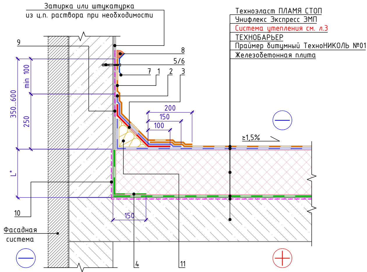
Спецификация на узел У.2.1-2021.03
