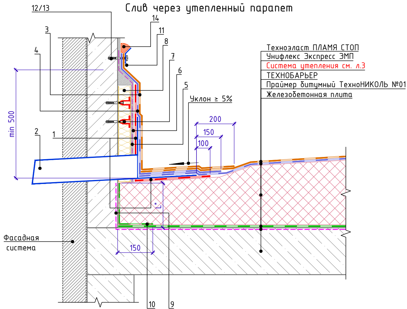
Спецификация на узел У.1.4-2021.03
