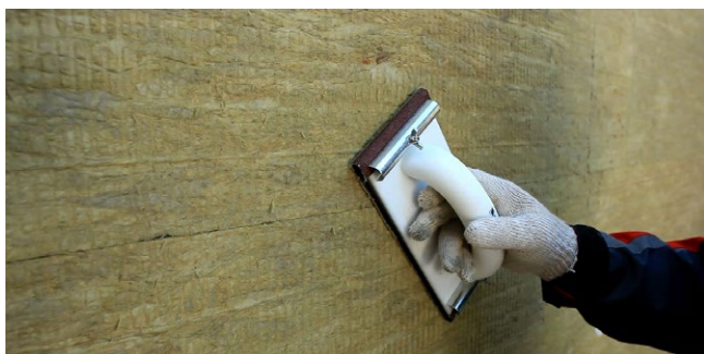
Рис. 32. Шлифовка стыков плит теплоизоляции наждачной бумагой
