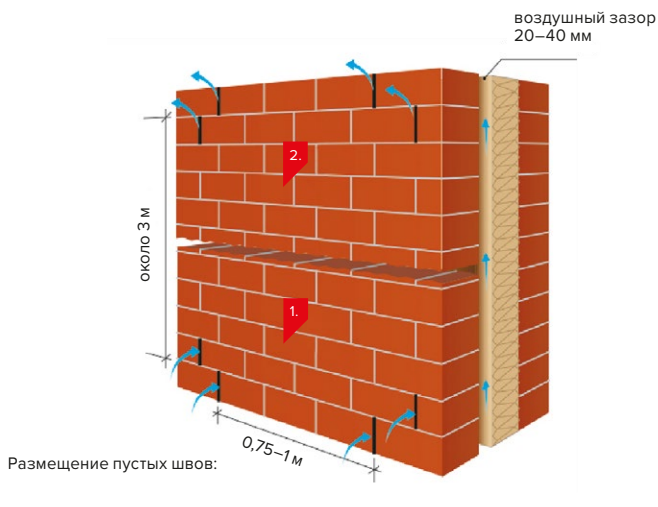
Рис. 17. Обеспечение притока и оттока воздуха при помощи продухов в конструкции слоистой кладки
