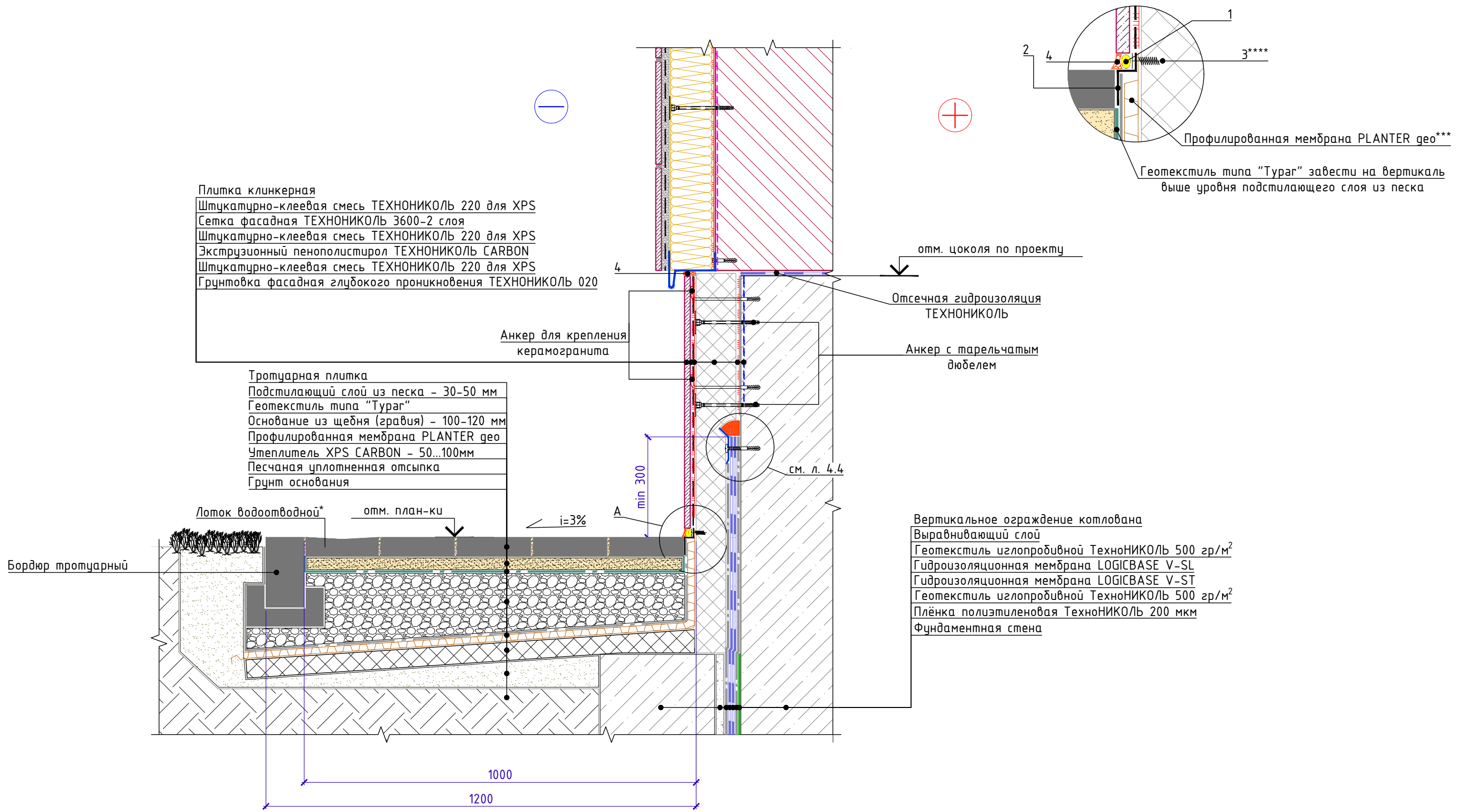
Спецификация на узел У.4.1-2020.11
