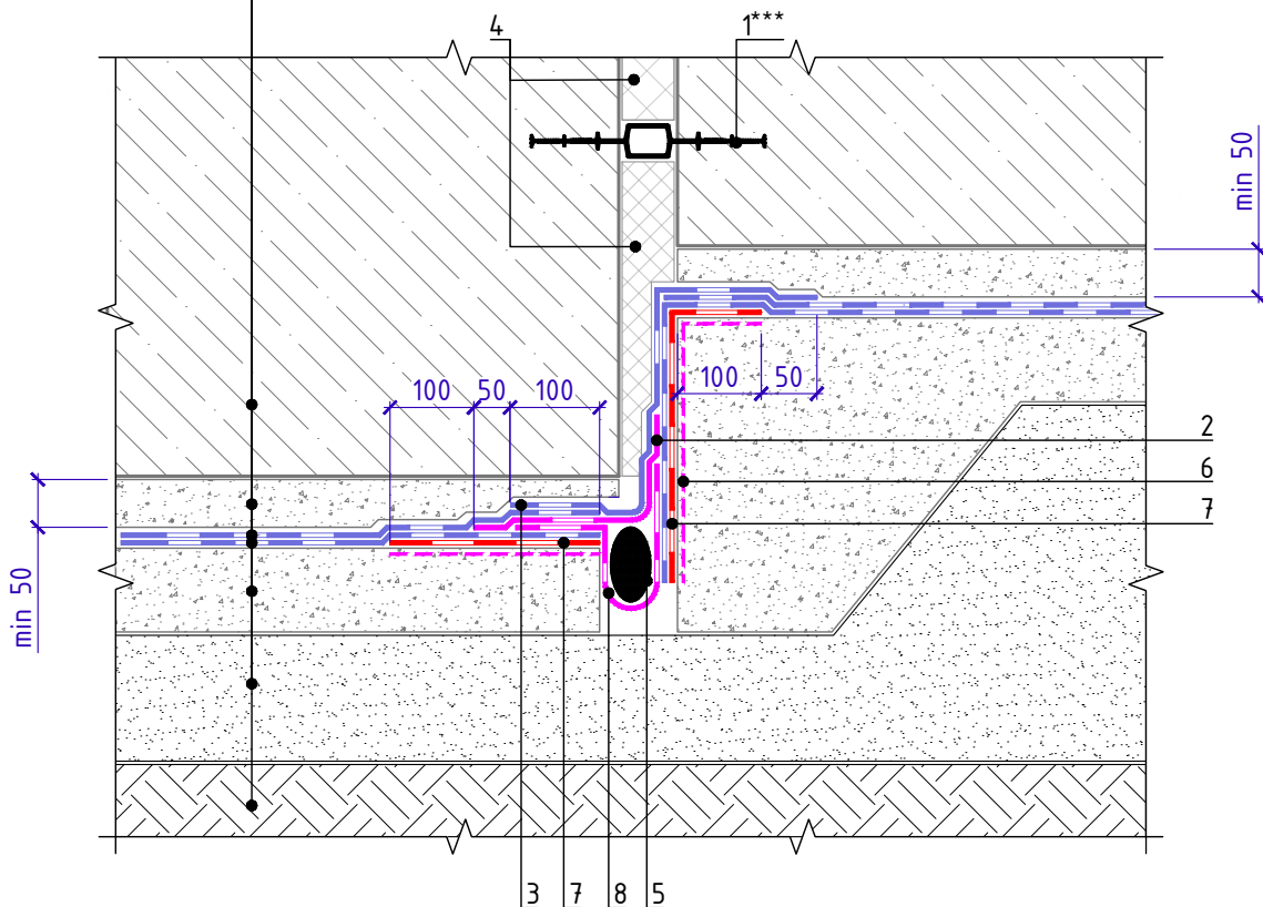
Спецификация на узел Ч.3.3-2023.04
