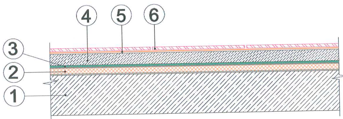
Рис. 2. Схема конструктивного исполнения железобетонного междуэтажного перекрытия с утепленным полом "ТН-ПОЛ Стандарт" (вариант 2)
