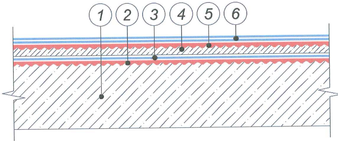
Рис. 14. Схема конструктивного исполнения железобетонного междуэтажного перекрытия с гидроизоляцией "ТН-ПОЛ ТАЙКОР Барьер" (вариант 14)
