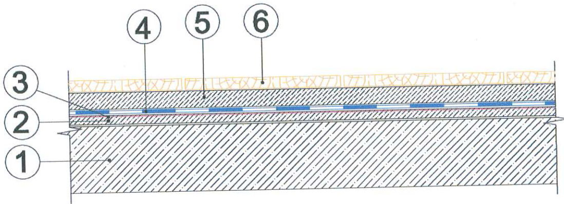
Рис. 3. Схема конструктивного исполнения железобетонного междуэтажного перекрытия с полом типа "ТН-ПОЛ Барьер" (вариант 3)
