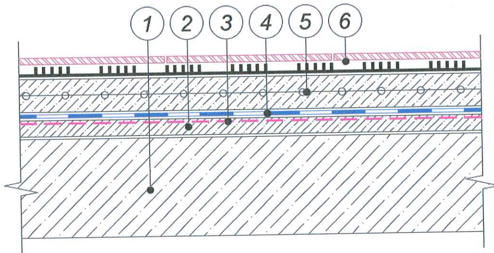
Рис. 3.2. Схема конструктивного исполнения железобетонного междуэтажного перекрытия с полом типа "ТН-ПОЛ Барьер" (вариант 3.2.)
