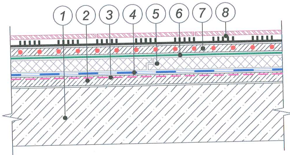
Рис. 3.1. Схема конструктивного исполнения железобетонного междуэтажного перекрытия с утепленным полом типа "ТН-ПОЛ Барьер" (вариант 3.1.)
