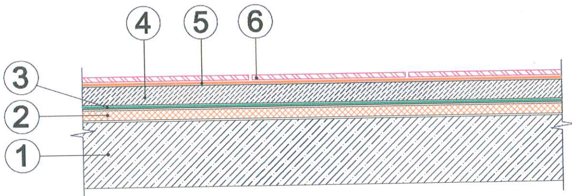
Рис. 9. Схема конструктивного исполнения железобетонного междуэтажного перекрытия с утепленным полом ТН-ПОЛ Термо PIR (вариант 9)
