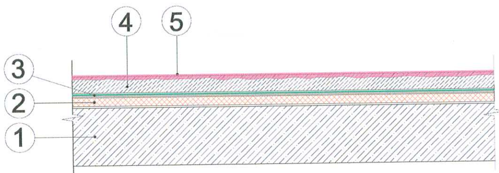
Рис. 10. Схема конструктивного исполнения железобетонного междуэтажного перекрытия с утепленным полом "ТН-ПОЛ ТАЙКОР Лайт" (вариант 10)
