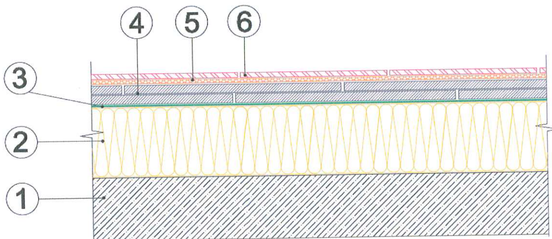
Рис. 5. Схема конструктивного исполнения железобетонного междуэтажного перекрытия с утепленным полом типа "ТН-ПОЛ Проф" (вариант 5)
