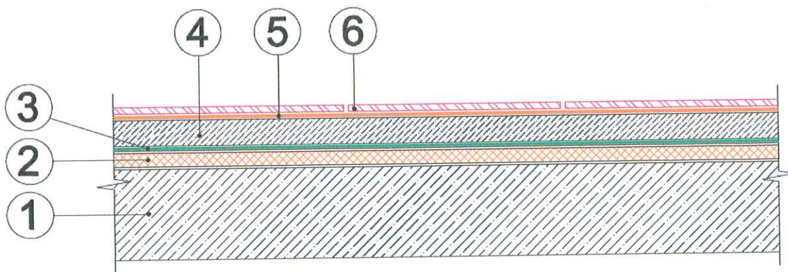
Рис. 4. Схема конструктивного исполнения железобетонного междуэтажного перекрытия с утепленным полом типа "ТН-ПОЛ Термо" (вариант 4)
