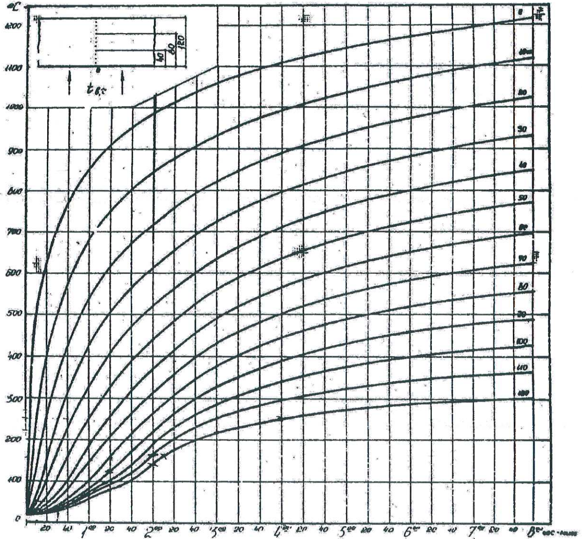
Рис. 1. Данные по прогреву необогреваемой поверхности бетонных плит толщиной 10-120 мм плотностью 2330 кг/м 3 и влажностью 2,0 % на гранитном заполнителе при одностороннем тепловом воздействии по стандартному температурному режиму
