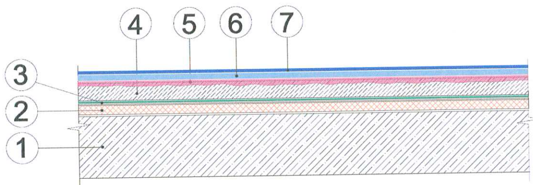
Рис. 11. Схема конструктивного исполнения железобетонного междуэтажного перекрытия с утепленным полом "ТН-ПОЛ ТАЙКОР Декор" (вариант 11)
