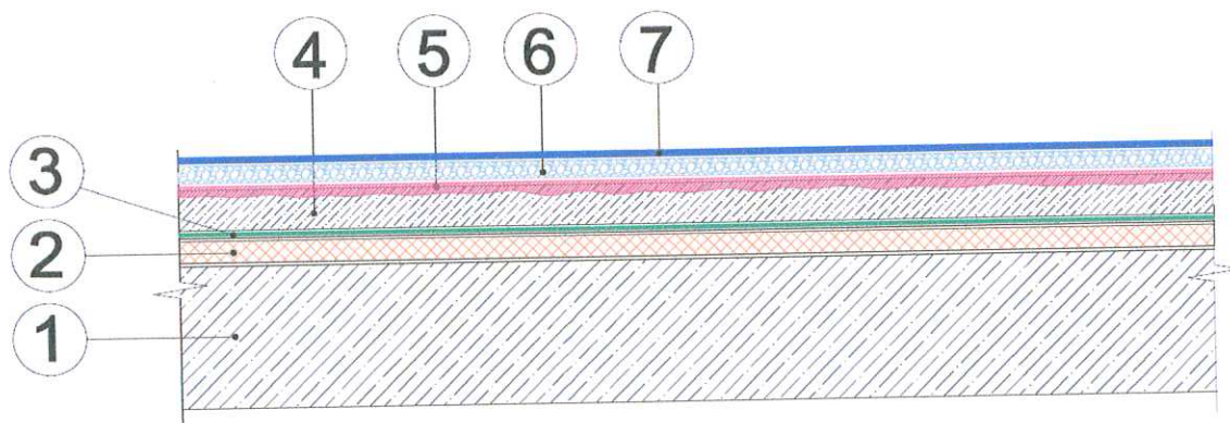
Рис. 13. Схема конструктивного исполнения железобетонного междуэтажного перекрытия с утепленным полом "ТН-ПОЛ ТАЙКОР Кварц" (вариант 13)
