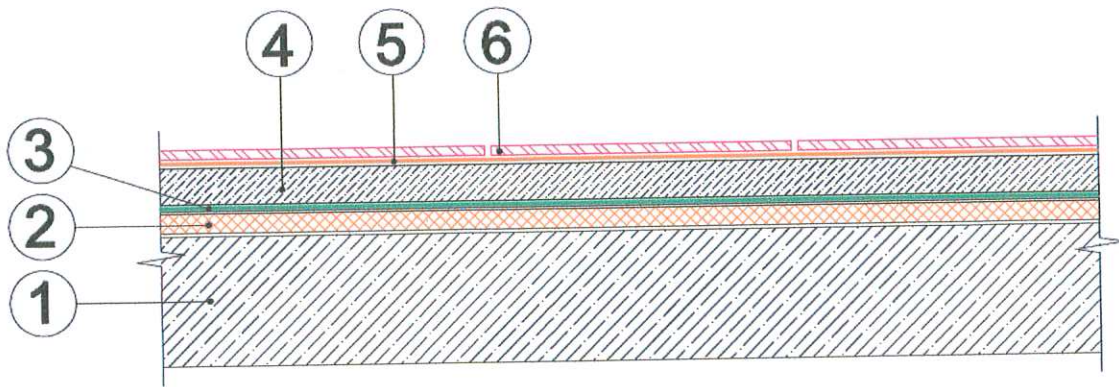
Рис. 8. Схема конструктивного исполнения железобетонного междуэтажного перекрытия с утепленным полом ТН-ПОЛ Стандарт PIR (вариант 8)
