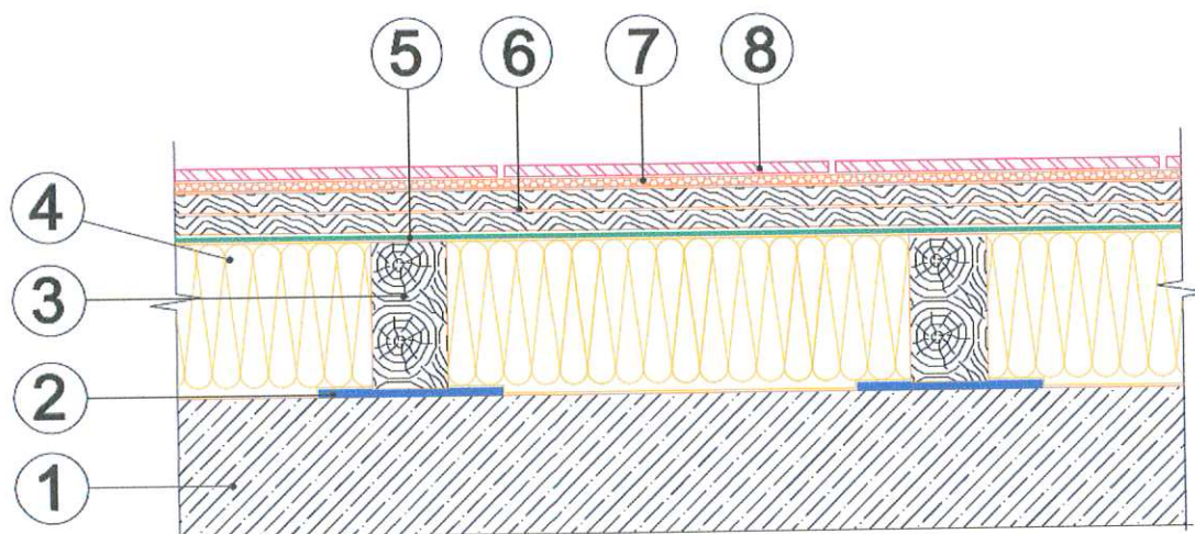
Рис. 7. Схема конструктивного исполнения железобетонного междуэтажного перекрытия с утепленным полом (вариант 7)
