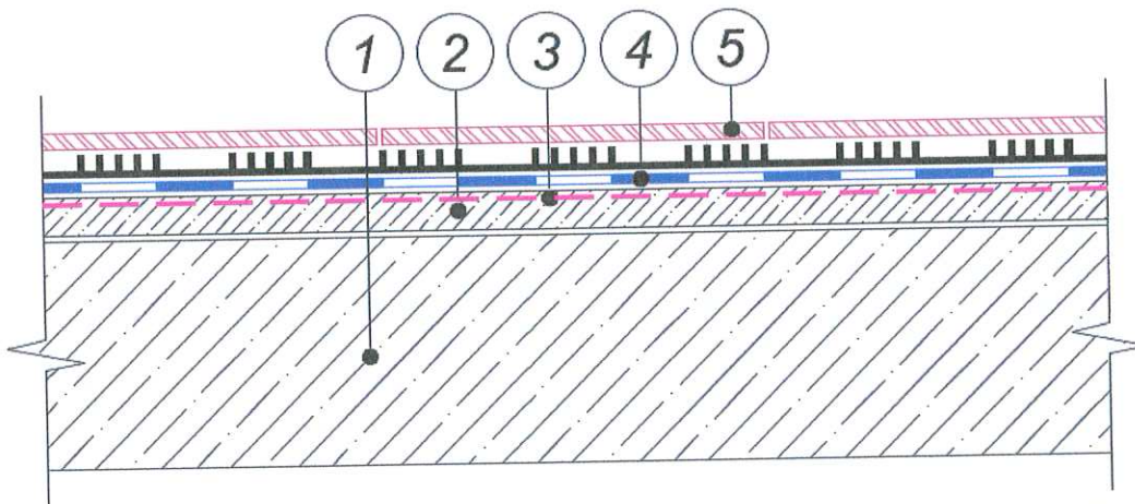
Рис. 3.3. Схема конструктивного исполнения железобетонного междуэтажного перекрытия с полом типа "ТН-ПОЛ Барьер Лайт" (вариант 3.3.)
