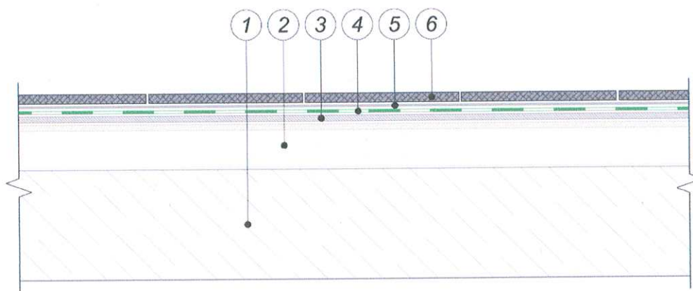
Рис. 16. Схема конструктивного исполнения железобетонного междуэтажного перекрытия с утеплением пола теплоизоляционными сэндвич-панелями на основе экструзионного пенополистирола ТЕХНОНИКОЛЬ Ц-ХПС (вариант 16)
