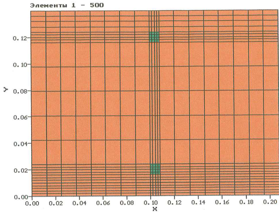
Рис. 18. Конечно-элементное разбиение конструкции для решения теплотехнической задачи
