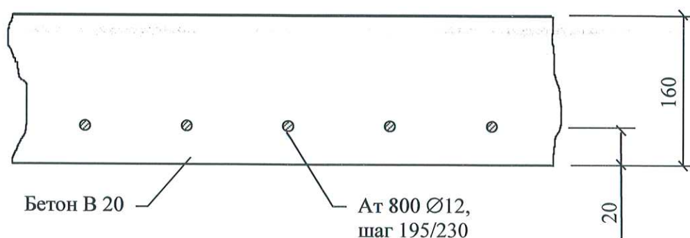
Рис. 17. Расчетное сечение конструкции
