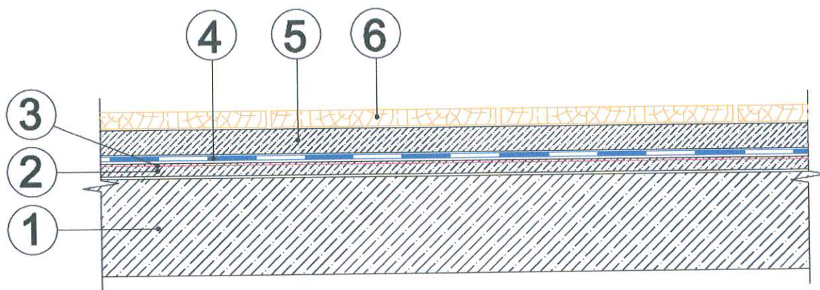
Рис. 6. Схема конструктивного исполнения железобетонного междуэтажного перекрытия с утепленным полом типа "ТН-ПОЛ Маст" (вариант 6)
