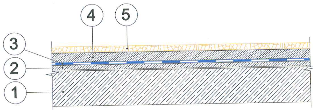
Рис. 1. Схема конструктивного исполнения железобетонного междуэтажного перекрытия с полом типа "ТН-ПОЛ Акустик" (вариант 1)
