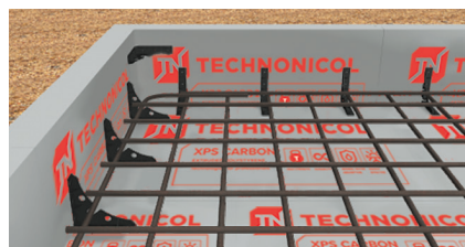
Плитный фундамент
