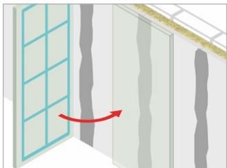
Рис. 15. Крепление листов ГКЛ/ГВЛ второго слоя
