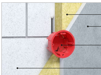
Рис. 18 а. Вариант монтажа электропроводки в несущей стене и подрозетника без дополнительной защиты
