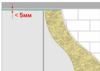
Рис. 13. Монтажный зазор
