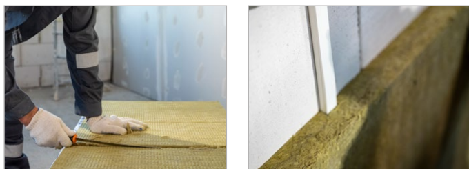
Рис. 9. Вырезанные борозды в плитах каменной ваты под кабель-канал
