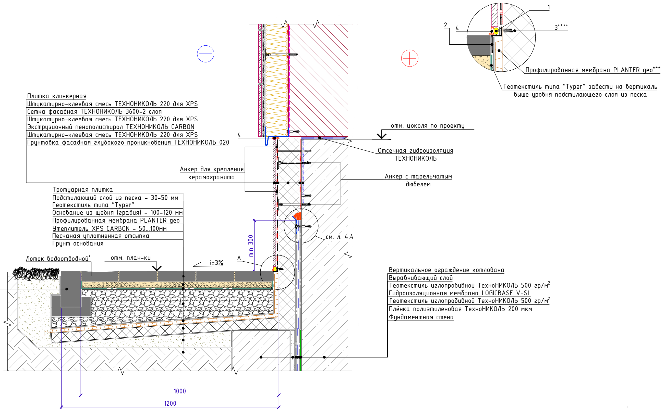
Спецификация на узел У.4.1-2020.11
