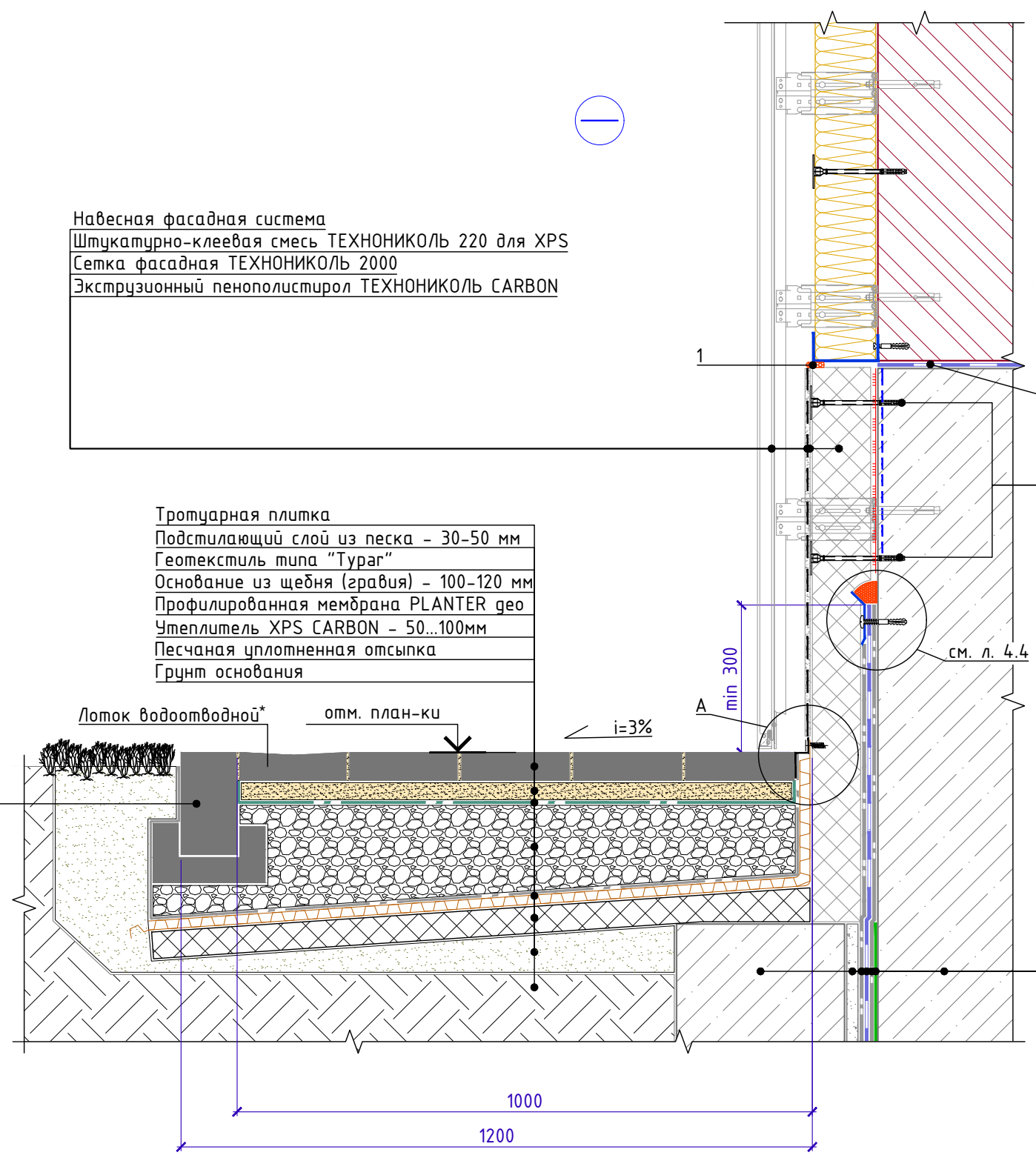
Спецификация на узел У.4.3-2020.11
