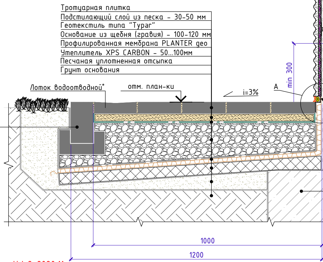
Спецификация на узел Ч.4.2-2020.11
