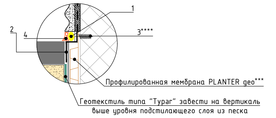
Узел А
