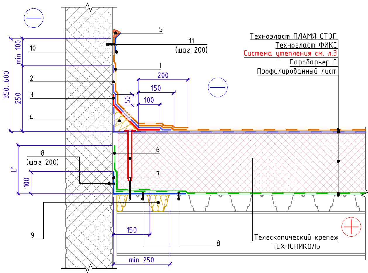
Спецификация на узел Ч.3.1-2020.08
