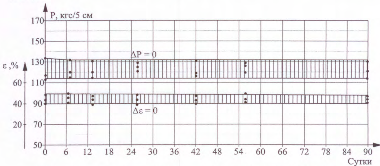
Рис. 2. Изменение прочности (1) и относительного удлинения (2) образцов рулонного материала "Техноэластмост Б" при воздействии 15-% раствора H_2SO_4
