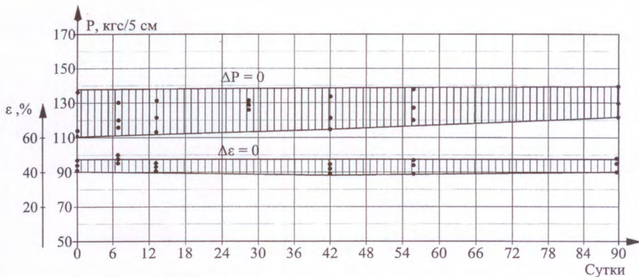
Рис. 1. Изменение прочности (1) и относительного удлинения (2) образцов рулонного материала "Техноэластмост Б" при воздействии 15-% раствора NaOH
