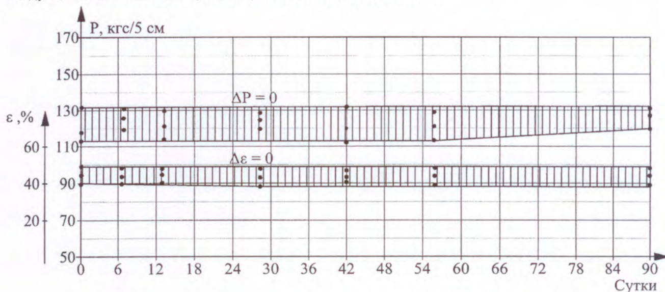
Рис. 3. Изменение прочности (1) и относительного удлинения (2) образцов материала "Техноэластмост Б" при воздействии насыщенного раствора NaCl
